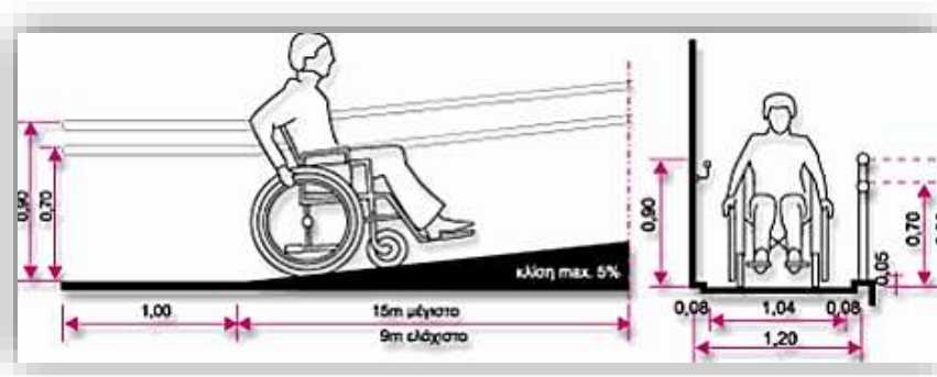
Εικόνα 59. Ράμπες Εισόδων (Υ.Π.ΕΝ., 2020)
