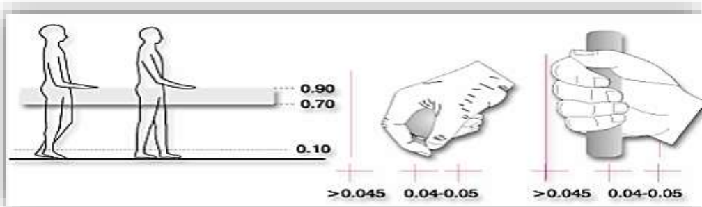
Εικόνα 60. Χειρολισθήρες (Υ.Π.ΕΝ., 2020)
