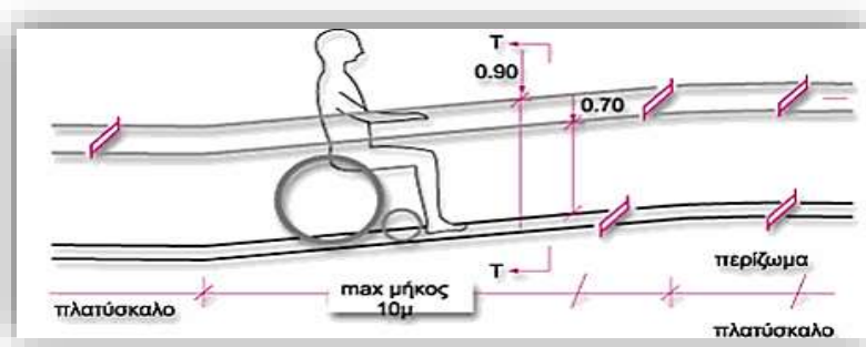
Εικόνα 58. Ράμπα (Υ.Π.ΕΝ., 2020)
